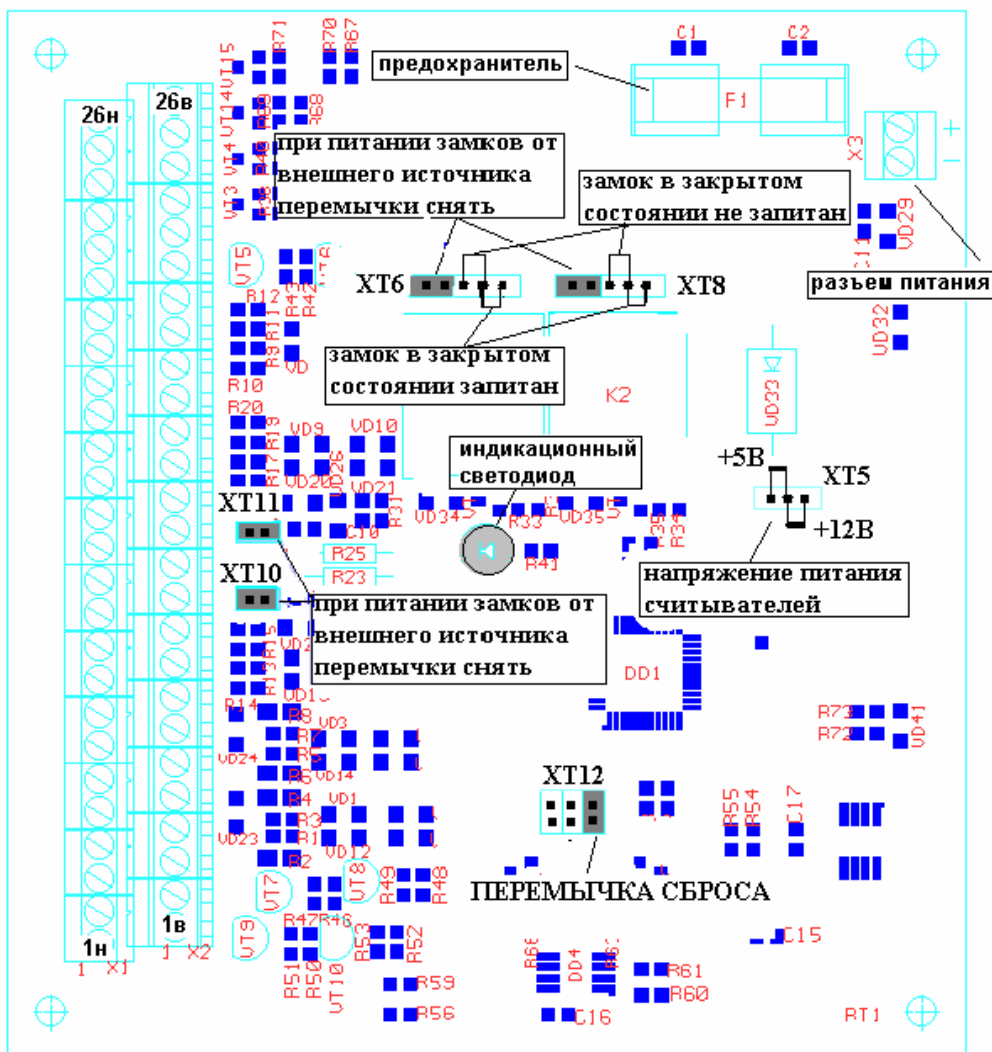
Рис. 1. Плата контроллера «Кронверк АТ-01».
