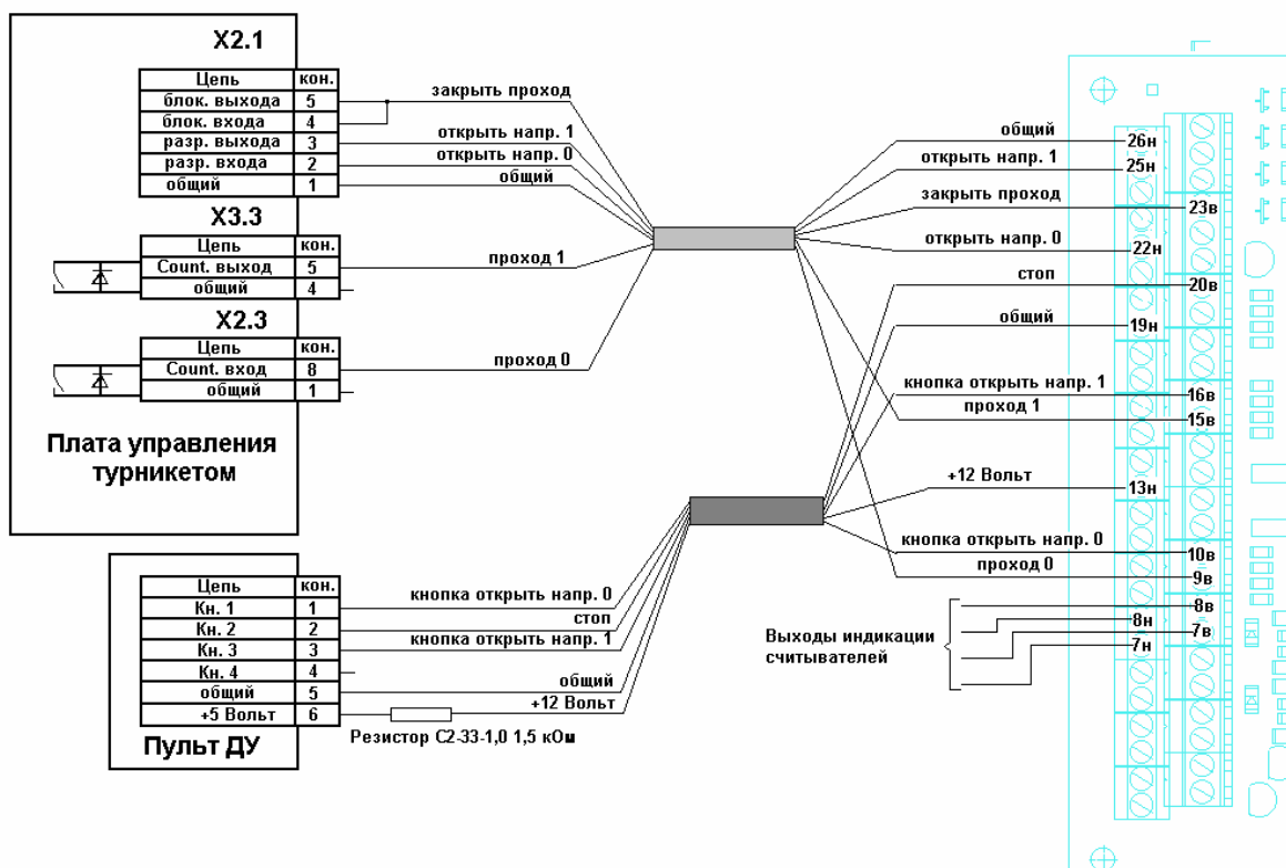
Рис. 11. Подключение турникета «Тrio™ Compact (ТТ1)».
