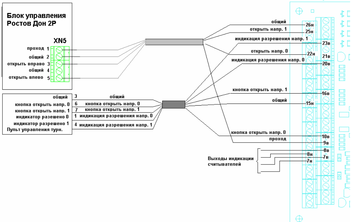
Рис.10. Подключение турникета «Ростов-Дон Р2».
