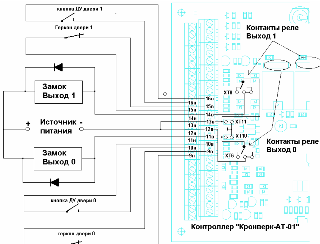
Рис.7. Подключение замков при использовании внешнего источника питания.
