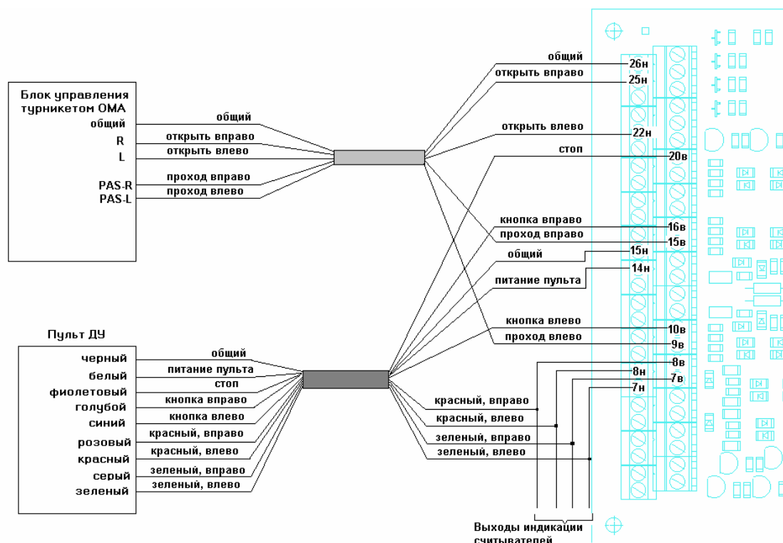
Рис.8 Подключение турникета фирмы «ОМА» к контроллеру «Кронверк АТ-01».
