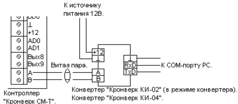
Рисунок 8.1.а: Подключение контроллера к компьютеру с использованием конвертера «Кронверк КИ-02»/«Кронверк КИ-04».
