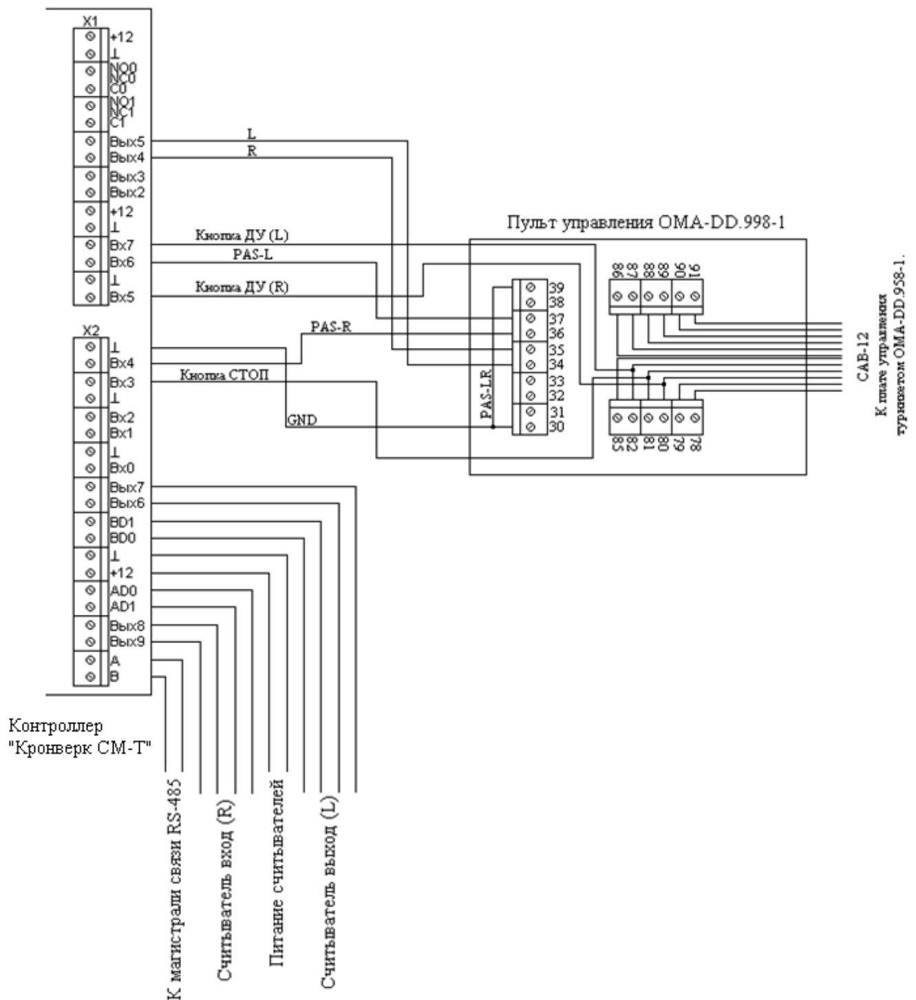
Рисунок 8.7: Схема подключения турникета "OMA" к контроллеру «Кронверк CM-T».
