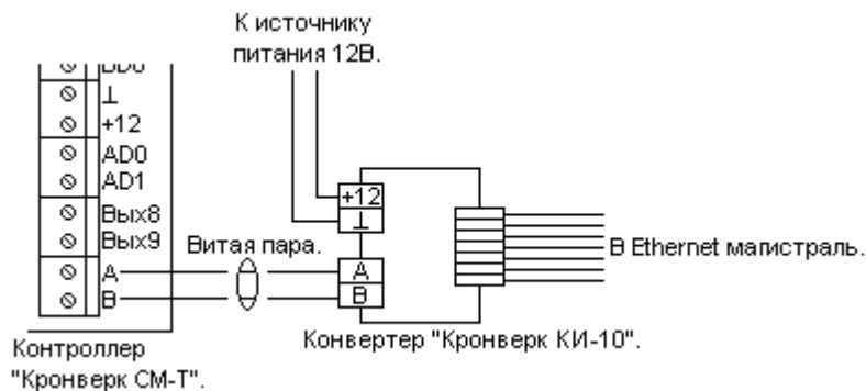
Рисунок 8.1.б: Подключение контроллера в локальную сеть с использованием конвертера «Кронверк КИ-10».
