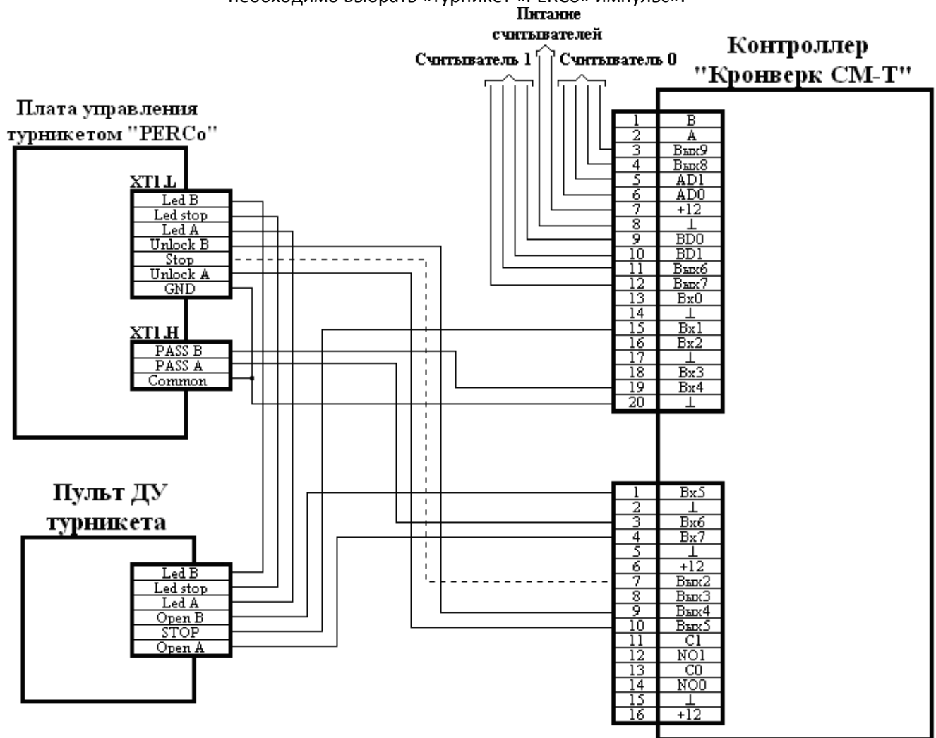
Рисунок 8.6: Подключение турникета "PERCo" к контроллеру «Кронверк SM-T».
