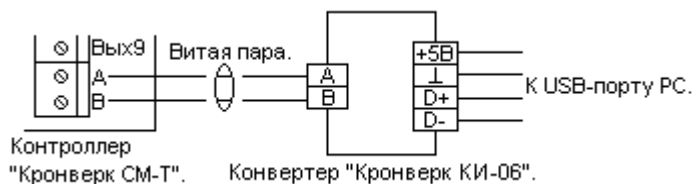
Рисунок 8.1.в: Подключение контроллера к компьютеру с использованием конвертера «Кронверк КИ-06».
