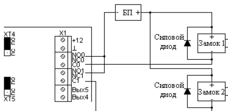
Рисунок 8.6.б: Подключение электромагнитных (электромеханических) замков, разблокирующегося подачей питания (контакты реле разомкнуты).
