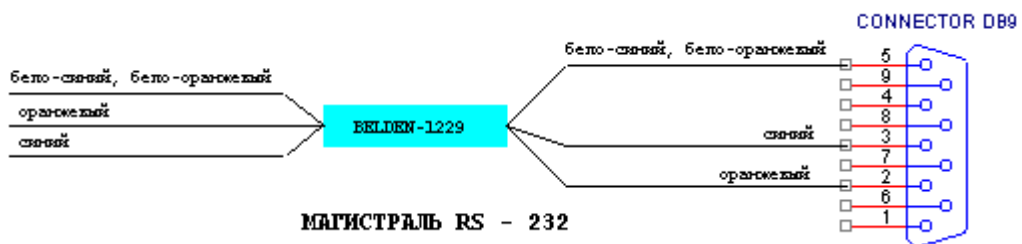
Рисунок 8.1. Кабель для подключения контроллера к компьютеру.
