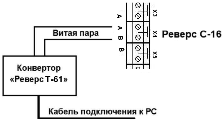
Рис. 8.2. Подключение одного контроллера «Реверс С16»
