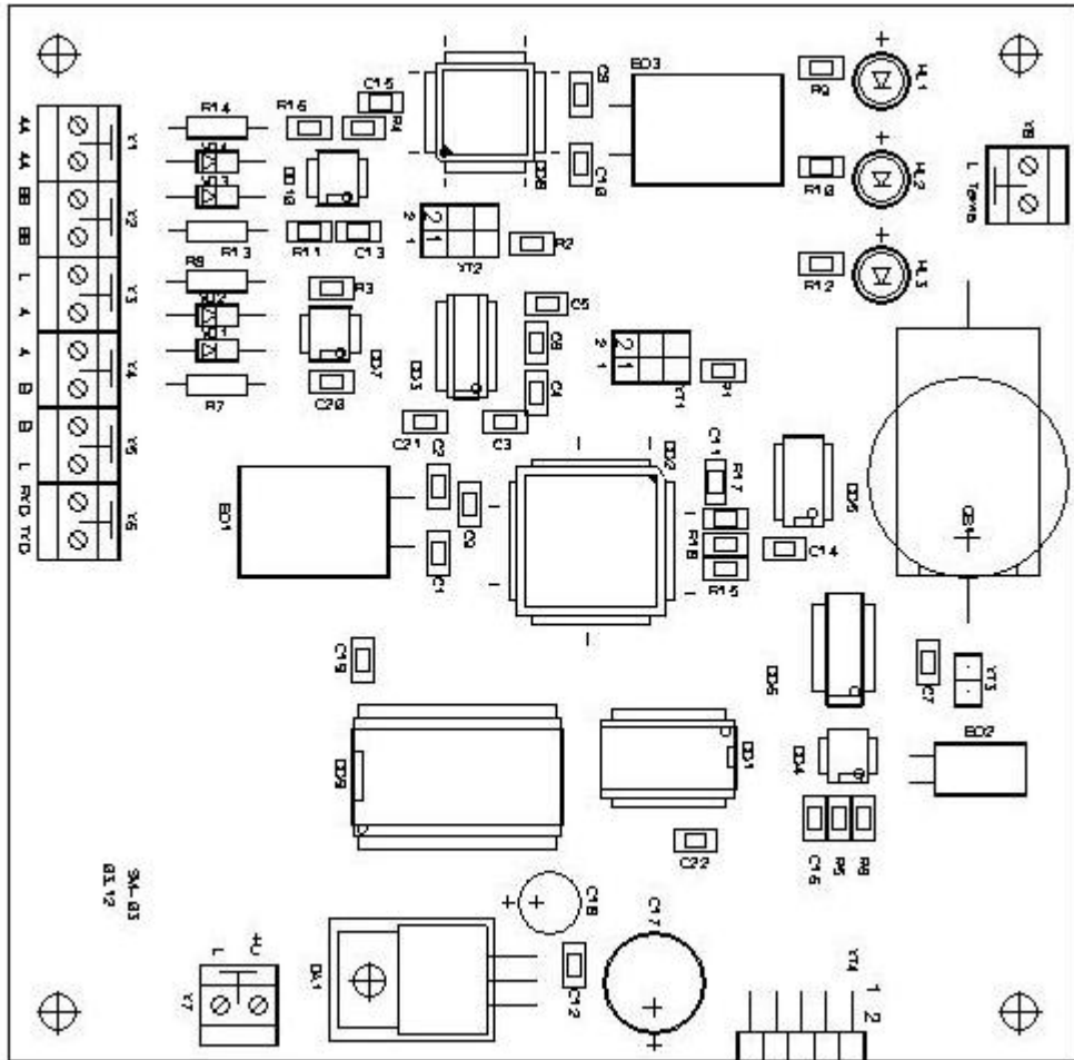
Рисунок 7.1 Плата контроллера "Реверс С16".
