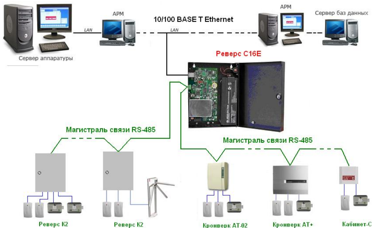
Рис.1 Структурная схема СКУД с использованием системного контроллера «Реверс С16Е»
