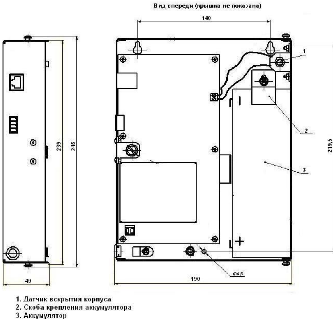
Рис.2. Габаритные и установочные размеры контроллера
